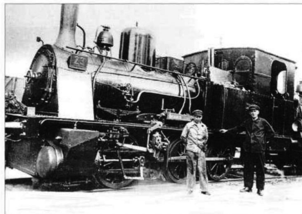
ASN-Lokomotive 23 wurde 1920 von Henschel geliefert und 1950 von der Deutschen Reichsbahn an die Maxhütte Unterwellenborn verkauft. Ihr letzter Einsatzort war das Stahl- und Walzwerk in Henningsdorf bei Berlin
