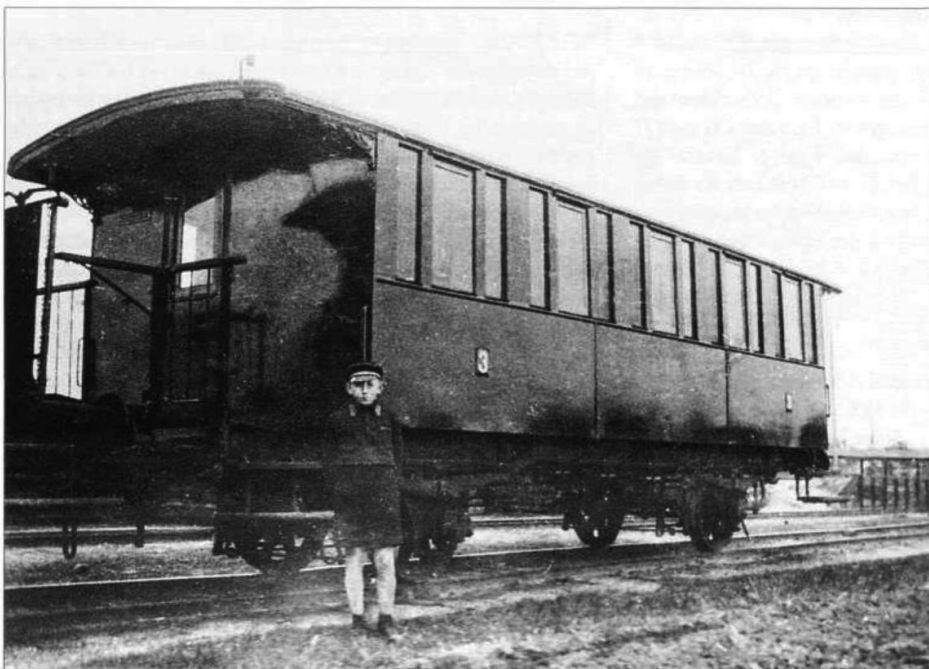
1940, im Jahr der Aufnahme, trug dieser Zweiachser die Nummer ASN 25. Er gehörte zur ersten Wagenserie, die Herbrandt 1896 an die ASN ausgeliefert hatte und war zunächst mit der Nummer 12 gekennzeichnet. Noch 1958 zählte das Fahrzeug zum Betriebspark der Deutschen Reichsbahn. Ob der junge Mann vor dem Wagen nur zu Erinnerung fotografiert wurde oder als angehender Eisenbahner, ist ebenso unbekannt wie sein Name
