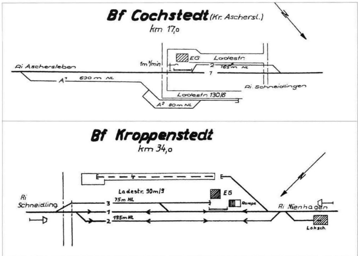
Gleispläne aus dem Jahr 1962; viel hatte sich gegenüber dem Betrieb in der Kleinbahnzeit nicht verändert
